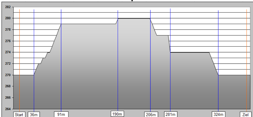
Höhenprofil
